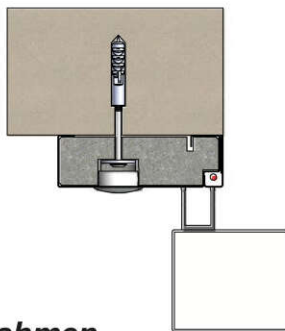
Flachrahmen Sacklochmontage
