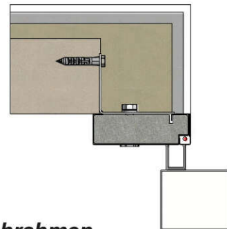
Flachrahmen Winkelmontage
