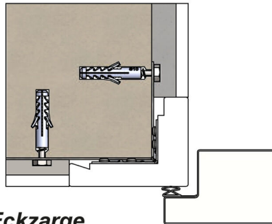
Rahmen für Eckzarge
