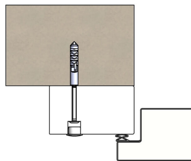
Flachrahmen 100 mm x 60 mm
